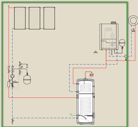
Abdeckung aller Systemkomponenten für das 100% ELCO System
